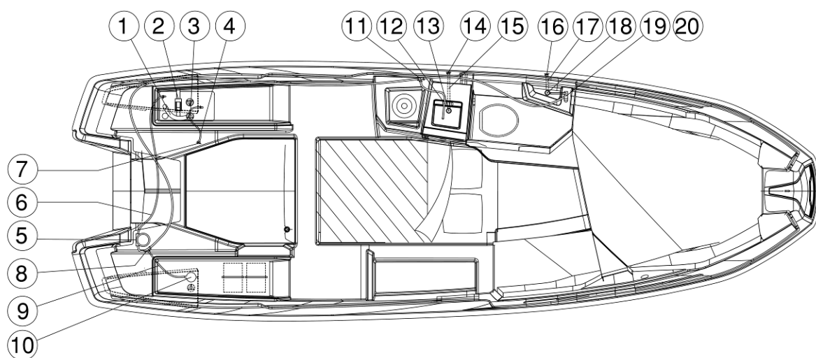
Bild: Färskvattensystem
