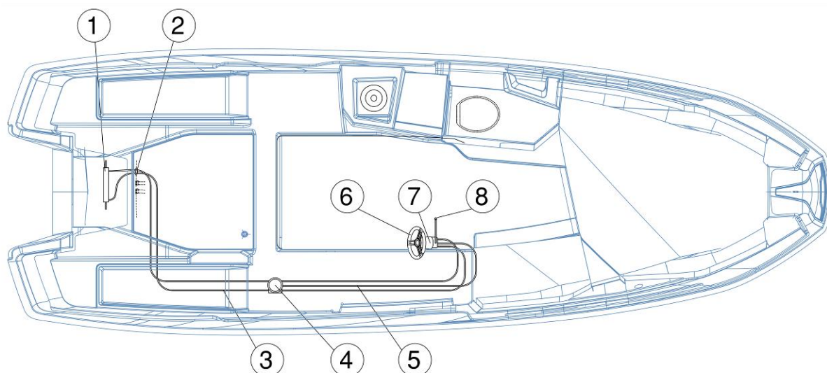
Bild: Styrsystem
