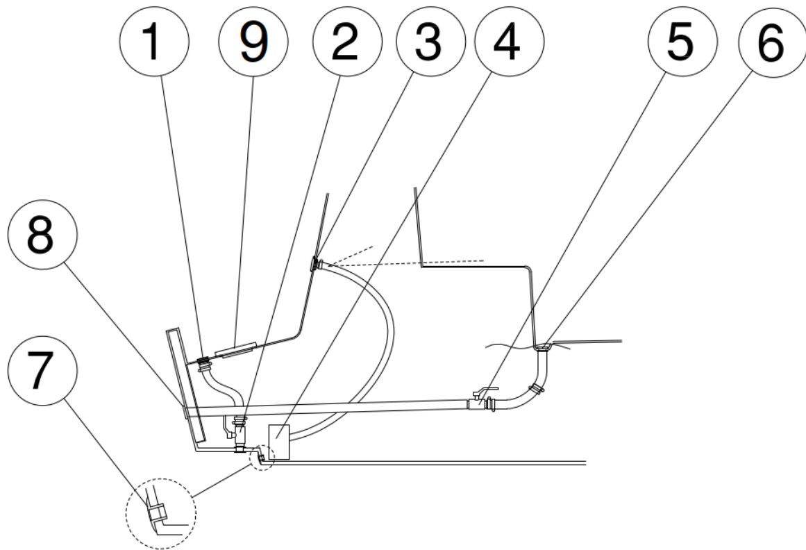
Kuva: Veneen tyhjennysjärjestelmä
