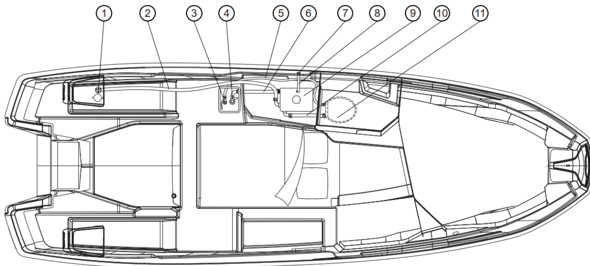
Kuva: Septijärjestelmä
